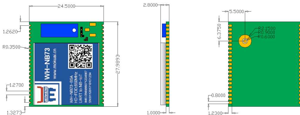
(NB73-B5/B8 尺寸图)
