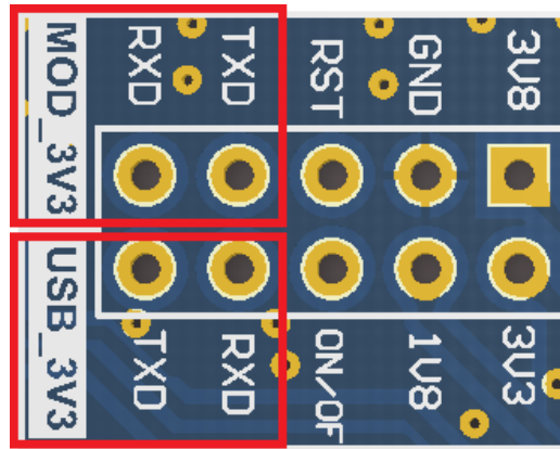
图 2 排针接口示意图
