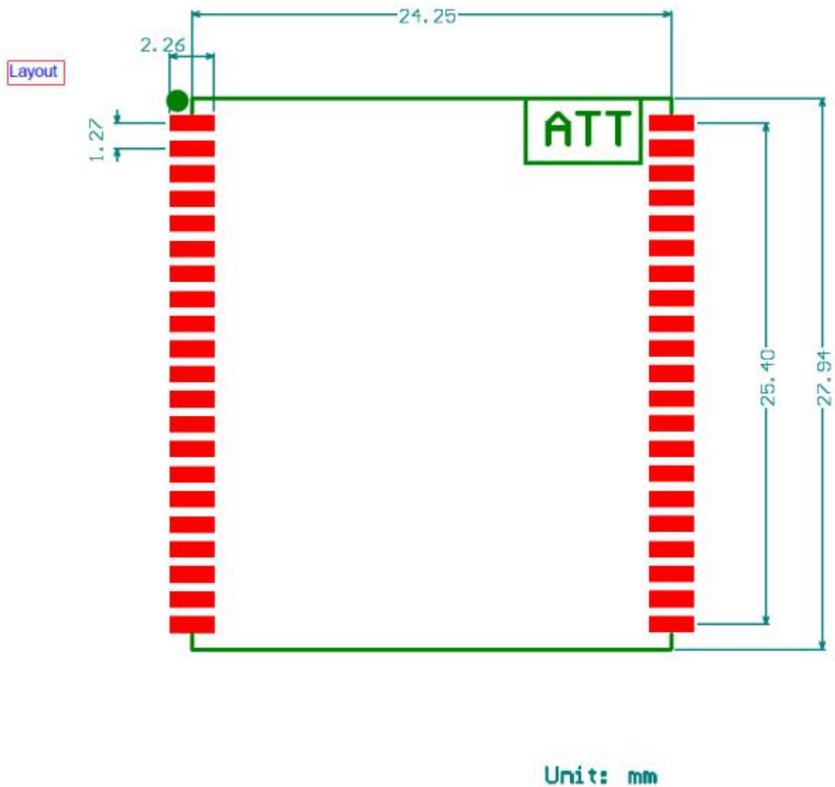
GM3/GM3s 焊盘封装尺寸
