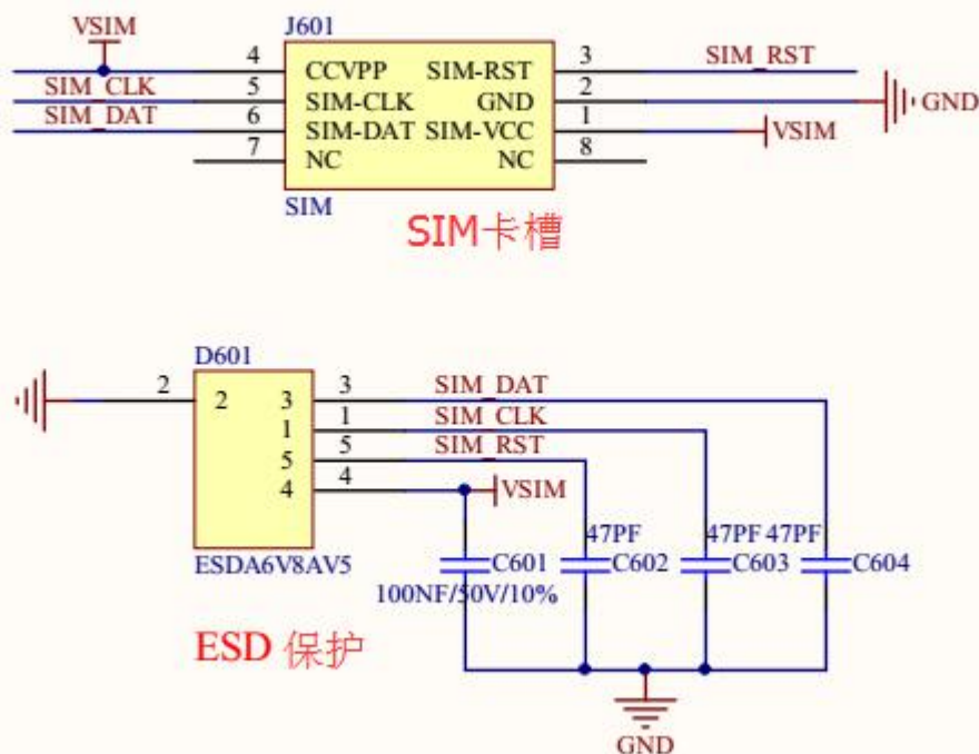
图 5-3 SIM 卡设计原理图
