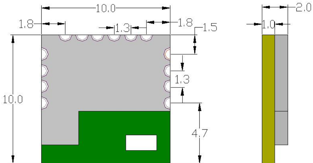
图 9. USR-BLE101 尺寸示意图
