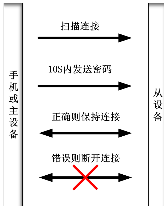
图 23. 密码配对验证流程图
