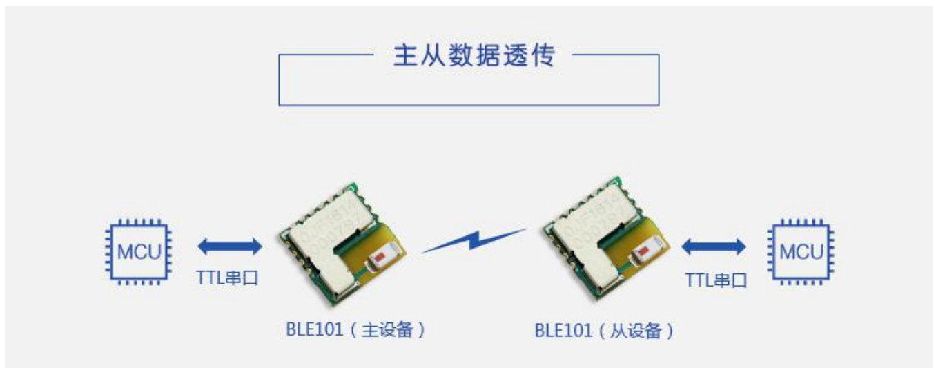
图 14. 主从数据透传示意图
