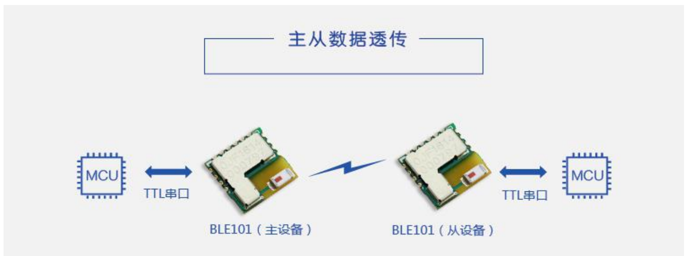
图 6. 主从数据透传示意图
