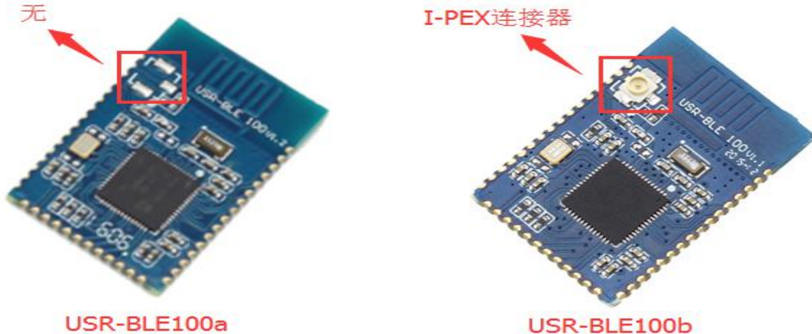
图 1. USR-BLE100a/USR-BLE100b 区别
