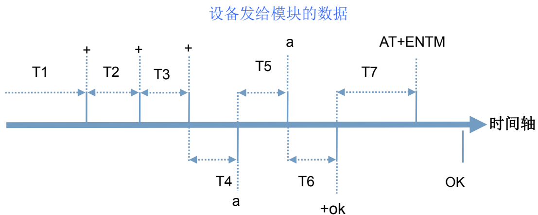
图 24. +++a 时序图
